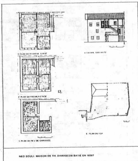
Σχέδιο 3. Κατοικία Θ. Λαμάσκου (1830)
