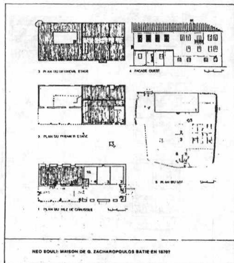
Σχέδιο 2. Κατοικία Γ. Ζαχαρόπουλου (1870)
