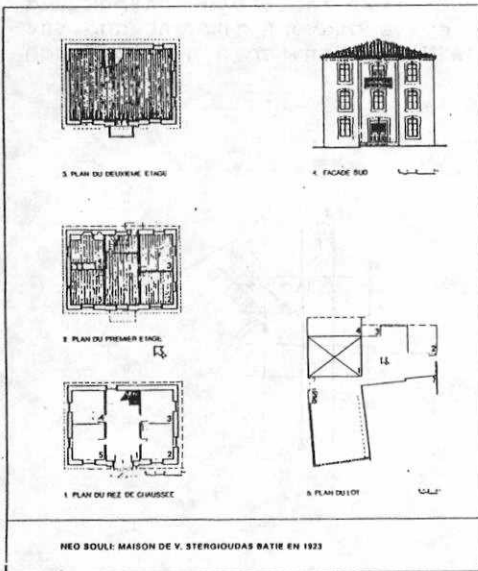
Σχέδιο 5. Κατοικία Β. Στεργιούδα (1923)
