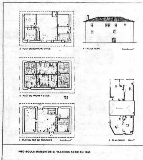
Σχέδιο 1. Κατοικία Γ. Βλάχου (1800)
